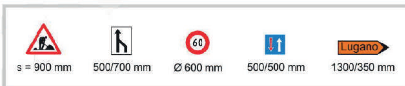
Signalgrösse im Normalformat Signaux de dimensions normales Segnale di dimensione normale
