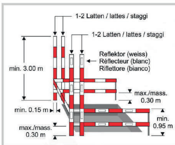
Abschränkungen im Baustellenbereich Barrières dans l'enceinte du chantier Delimitazioni in zona di cantiere
