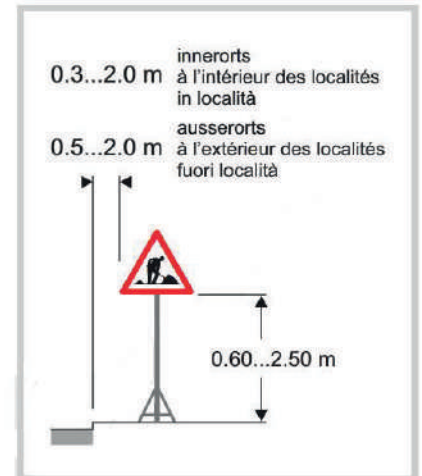
Abstand zum Fahrbahnrand Distance jusqu'au bord de la chaussée Distanza dal bordo della carreggiata
